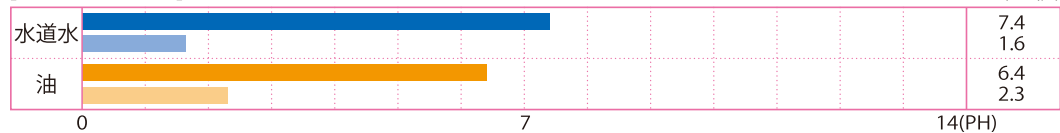
【テラヘルツ加工した分電盤】酸化測定グラフ(照射前・上段/照射30分後・下段)
